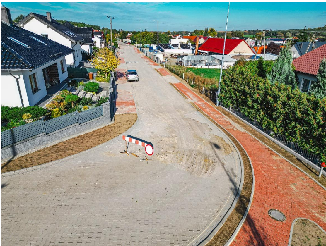
Budowa ulicy Zybera wraz z kanalizacją deszczową i oświetleniem w miejscowości Gostyń.
