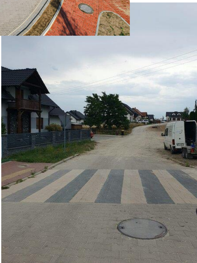
Budowa ulicy Zybera wraz z kanalizacją deszczową i oświetleniem w miejscowości Gostyń.
