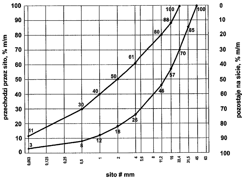
Rys. 1. Krzywe graniczne uziarnienia mieszanki mineralnej \emptyset /31,5 mm
